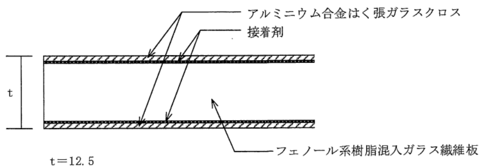
図 1 断面図
